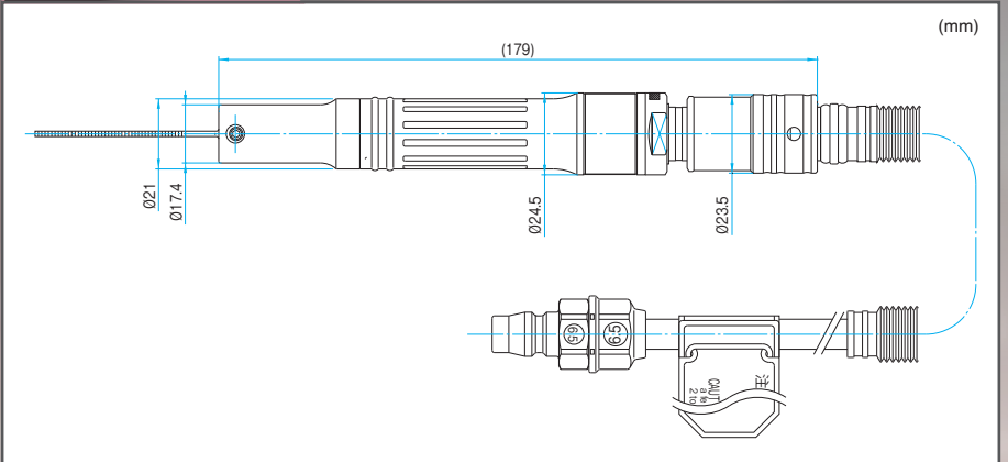
外観寸法図
