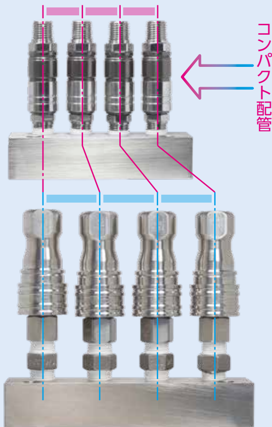
SPカブラ Type A (弊社製品)
